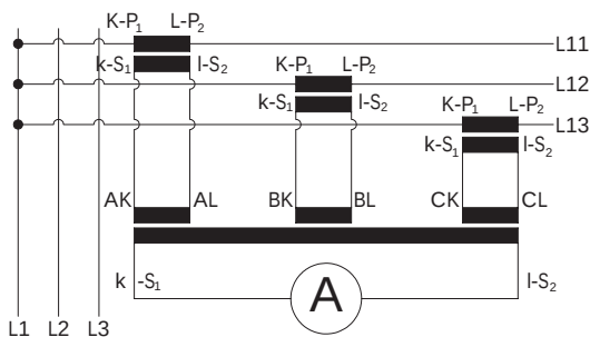
Summenwandler-Schaltung
