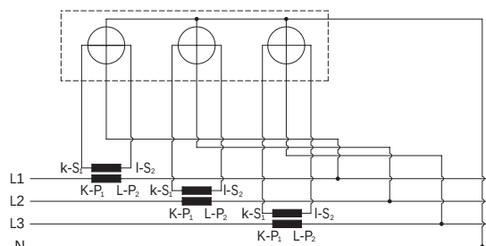
Zählerschaltung mehrphasig
