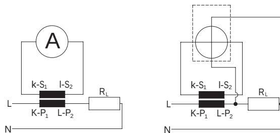
Meßschaltung
