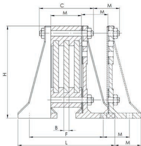
Abbildung 1 Beispiel eines unipolaren Schienenhalters mit 3 parallelen Schienenhaltern
