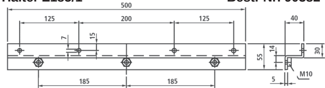
Halter Z185/2 (2 x M10 je Phase)
